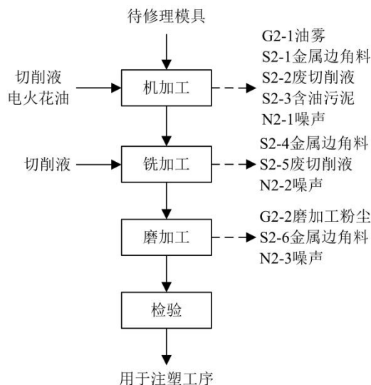
图 2-3 模具修理生产工艺流程图
