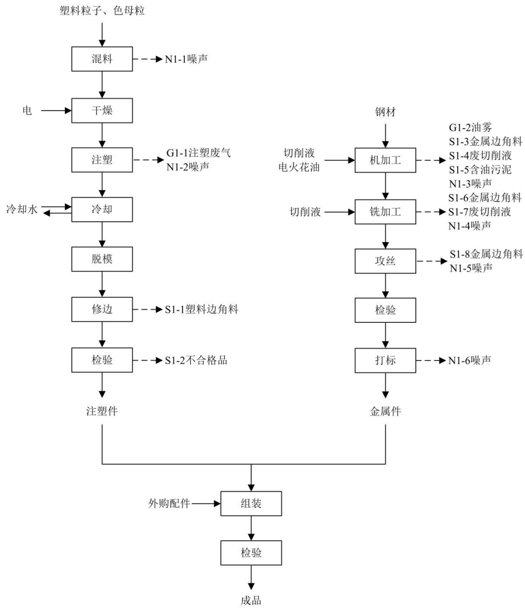
图 2-2 风叶轮生产工艺流程图
