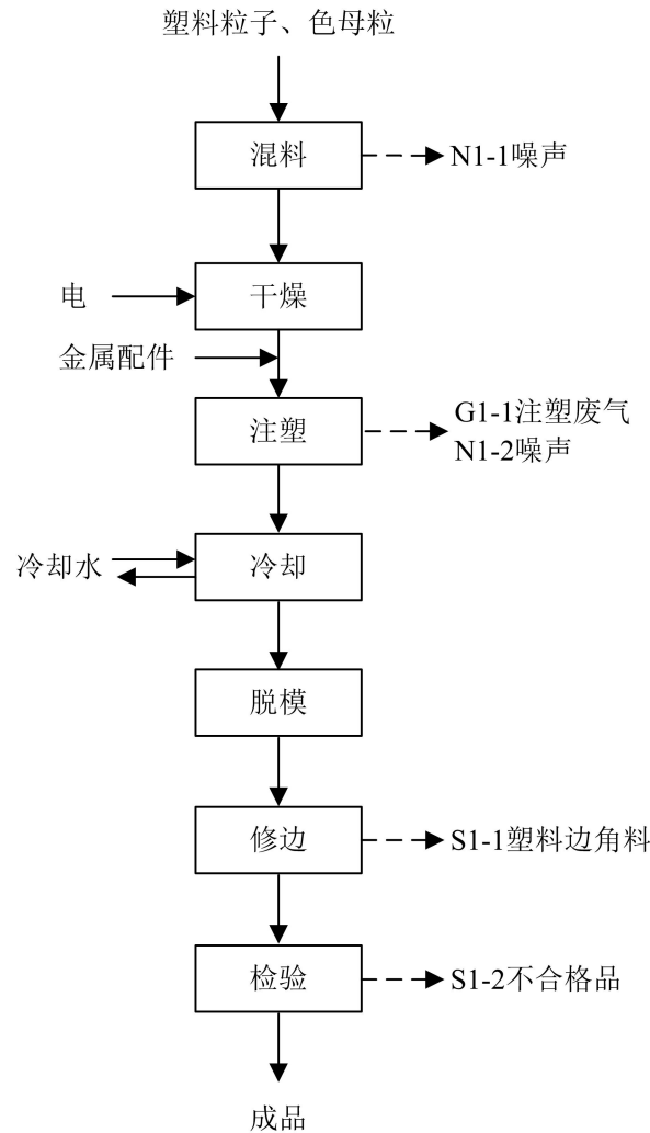
图 2-2 伺服电机配件生产工艺一流程图
