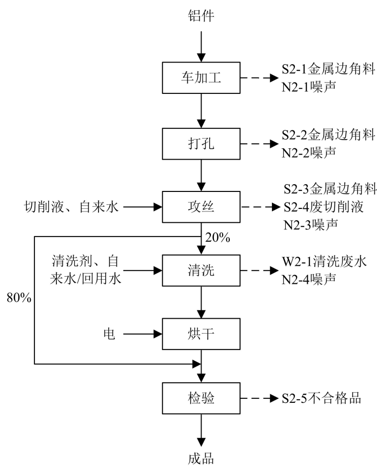
图 2-2 伺服电机配件生产工艺二流程图
