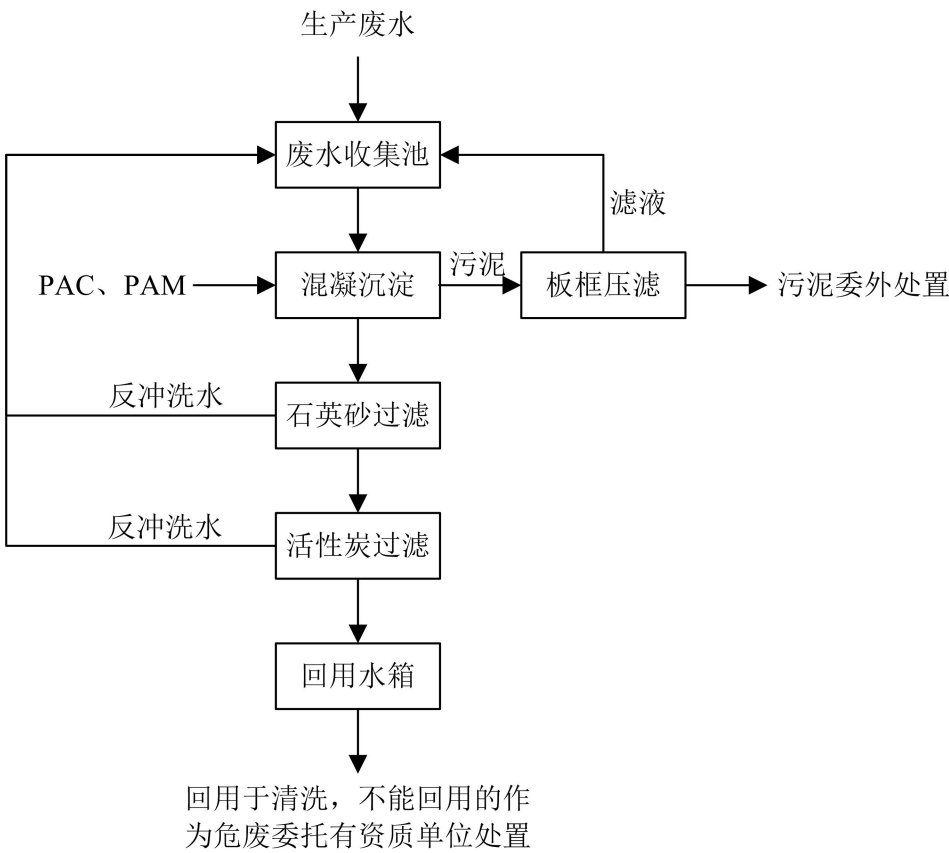
图 3-1 生产废水处理工艺流程图
