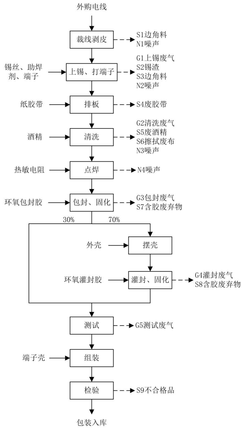
图 2-2 温度传感器生产工艺流程图
