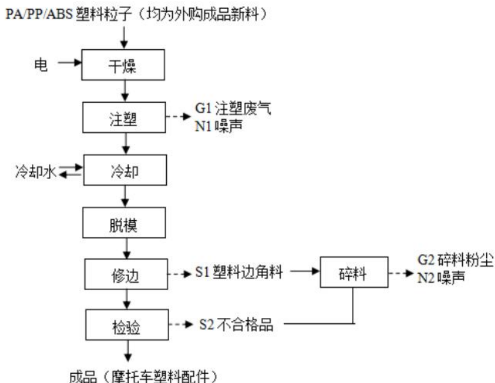
图 2-2 摩托车塑料配件生产工艺流程图
